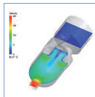
Simulación de la curva de velocidad en la cámara de turbulencia con CFD
