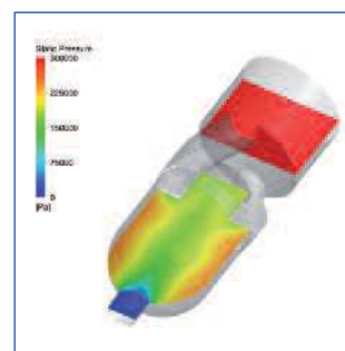
Simulación de presión estática en la cámara de turbulencia con CFD
