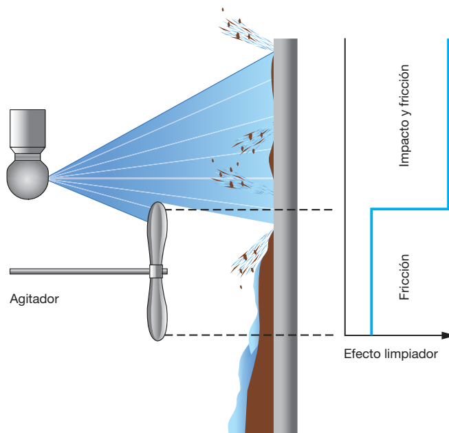
Ilustración 5. Mecanismos de limpieza, impacto y fricción
