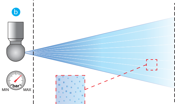
Ilustración 4. Toberas rotativas de limpieza trabajando con una presión demasiado elevada
